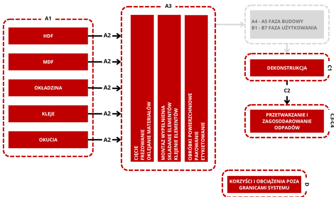
Rysunek 5.1: Granice systemu dla charakterystyki środowiskowej drzwi ramowych
