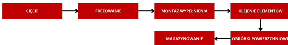
Rysunek 5.2: Uproszczony proces produkcji drzwi ramowych
